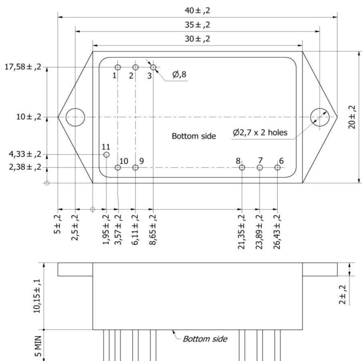
Одноканальное исполнение
