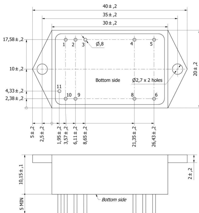
Двухканальное исполнение
